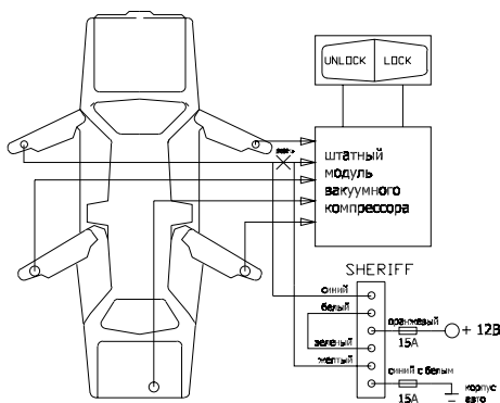
СХЕМА УПРАВЛЕНИЯ ДОПОЛНИТЕЛЬНЫМИ ЭЛЕКТРОПРОВОДАМИ
